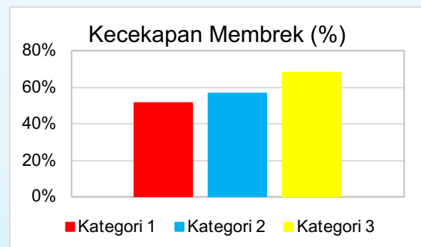
Rajah 2: Kecekapan membek bagi kenderaan kategori 1, 2 dan 3
