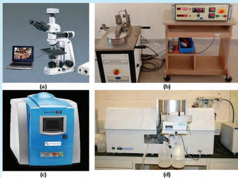
Rajah 2: Beberapa peralatan pengujian tribologi yang terdapat di Makmal STRIDE bagi mengdiagnosis punca kegagalan berasaskan kesan dari geseran, haus dan lusuh (a) Feroskop (b) Penguji pin on disc (c) Spectrometer elektrod cakera berputar (d) Spektrometer serapan atom
