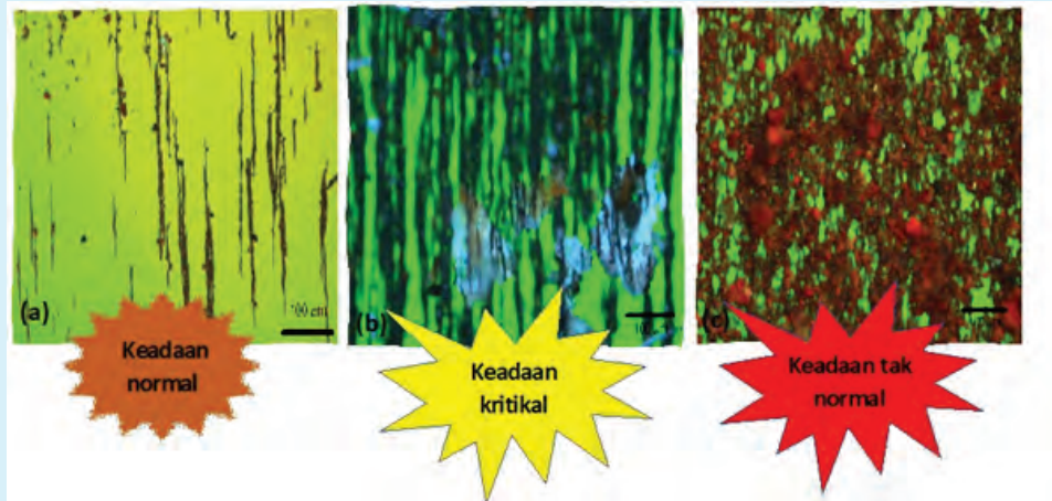
Rajah 1: Imej ferografik menunjukkan saiz partikel haus logam kurang dari 15 \mu\text{m} bagi (a) jentera utama (keadaan normal), lebih dari 50 \mu\text{m} bagi (b) janakuasa (keadaan kritikal) dan partikel berkepekatan tinggi bagi (c) kotak gear (keadaan tidak normal).
